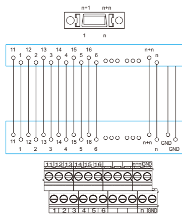
DM50-MDR-20-20-4Y-00A(H) DM50-MDR-26-26-4Y-00A(H) DM50-MDR-36-36-4Y-00A(H)
